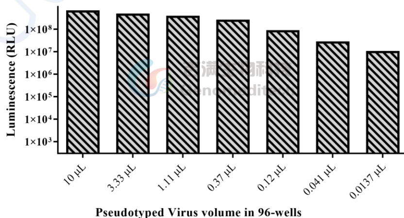
图2 吉满 SARS-CoV-2 Spike S 蛋白(BA.3.2)突变型假病毒感染 HEK293T-ACE2 测定 Luciferase 数值
