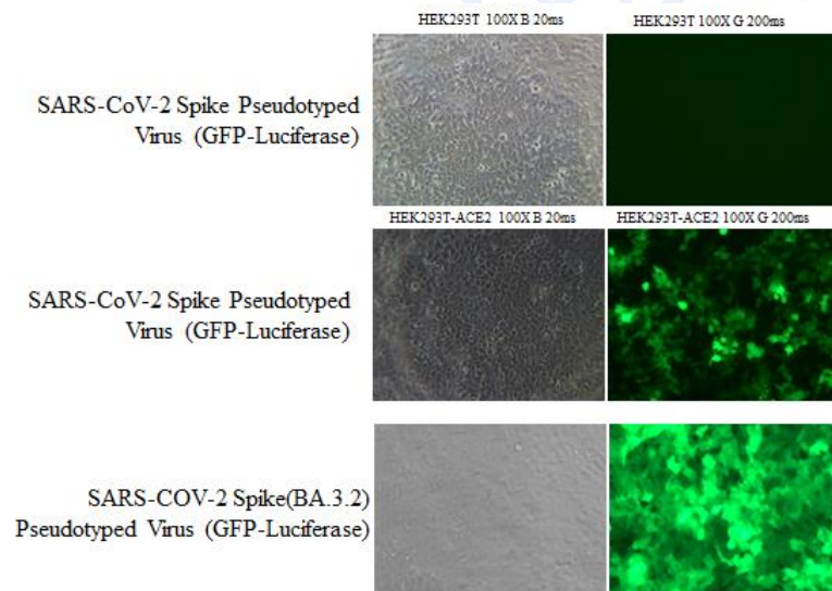
图1 SARS-CoV-2 Spike S 蛋白及突变型假病毒感染 HEK293 与 HEK293T-ACE2 荧光图片
